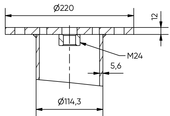
B-B ( 1 : 4 )
