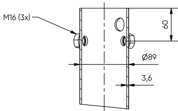
B-B ( 1 : 4 )
