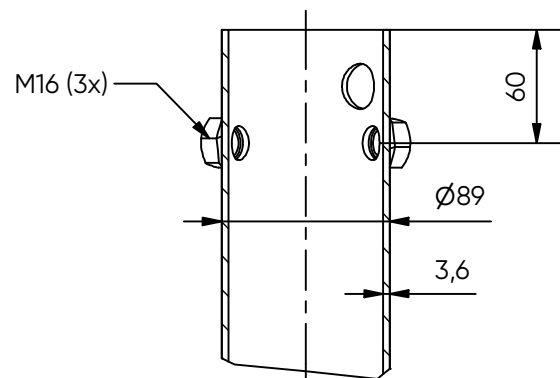
B-B (1 : 4)
