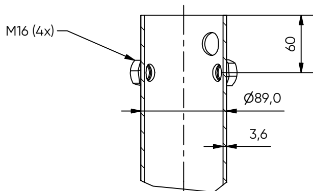
B-B ( 1 : 4 )
