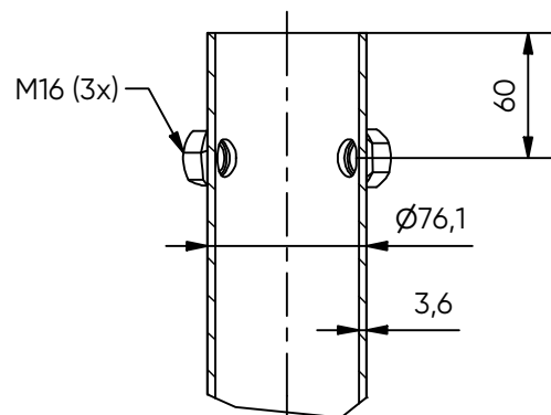
B-B ( 1 : 4 )
