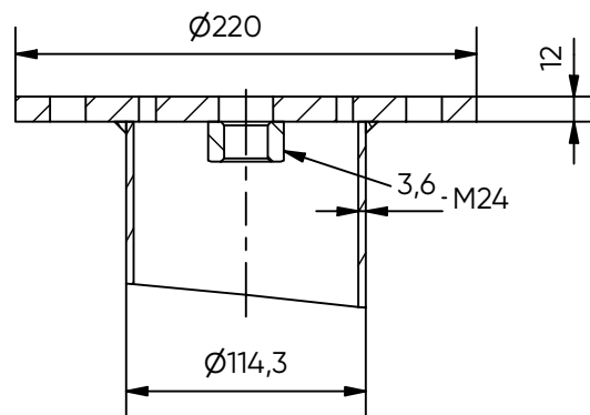
B-B ( 1 : 4 )
